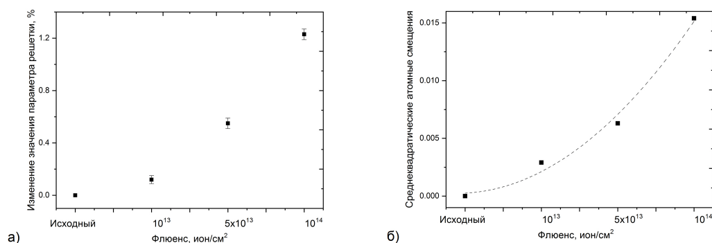
FIGURE 2 – Динамика изменения параметра кристаллической решетки (а) и величины среднеквадратичных смещений атомов (б) в процессе облучения
