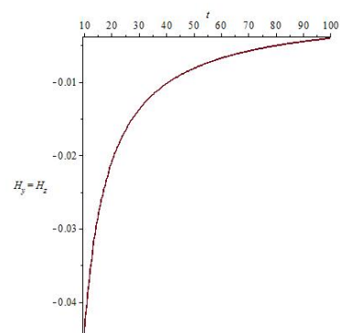
Сурет 5 – y және z бағытындағы H_y, H_z Хаббл параметрлерінің t уақытқа тәуелділік графигі. C_1 = 10, C_2 = -10, m = -3 .
