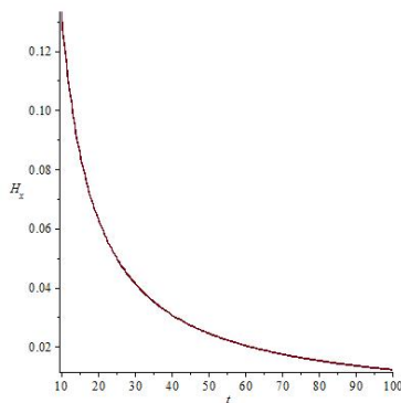
Сурет 4 – x бағытындағы H_x Хаббл параметрінің t уақытқа тәуелділік графигі. C_1 = 10, C_2 = -10, m = -3 .
