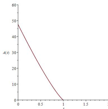
Сурет 2 – A масштабтық факторының t уақытқа тәуелділік графигі. C_1 = 10, C_2 = -10, m = -3 .
