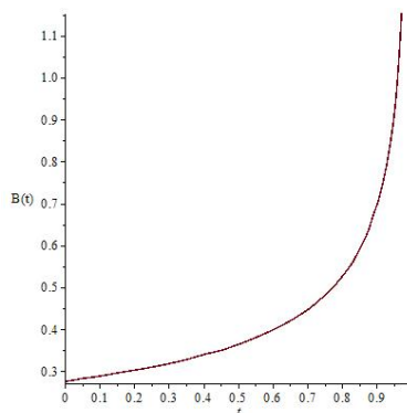
Сурет 1 – B масштабты факторының t уақытқа тәуелділік графигі. C_1 = 10, C_2 = -10, m = -3 .
