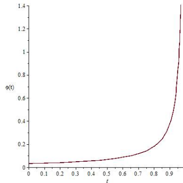
Сурет 3 – \phi скалярлық өрісінің t уақытқа тәуелділік графигі. C_1 = 10, C_2 = -10, m = -3, \alpha = -8 .
