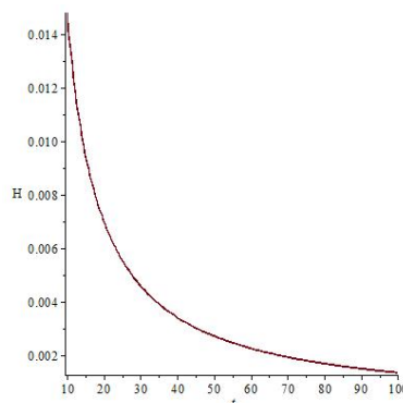
Сурет 6 – H Хаббл параметрінің жалпы түрінің t уақытқа тәуелділік графигі. C_1 = 10, C_2 = -10, m = -3, \alpha = -8 .
