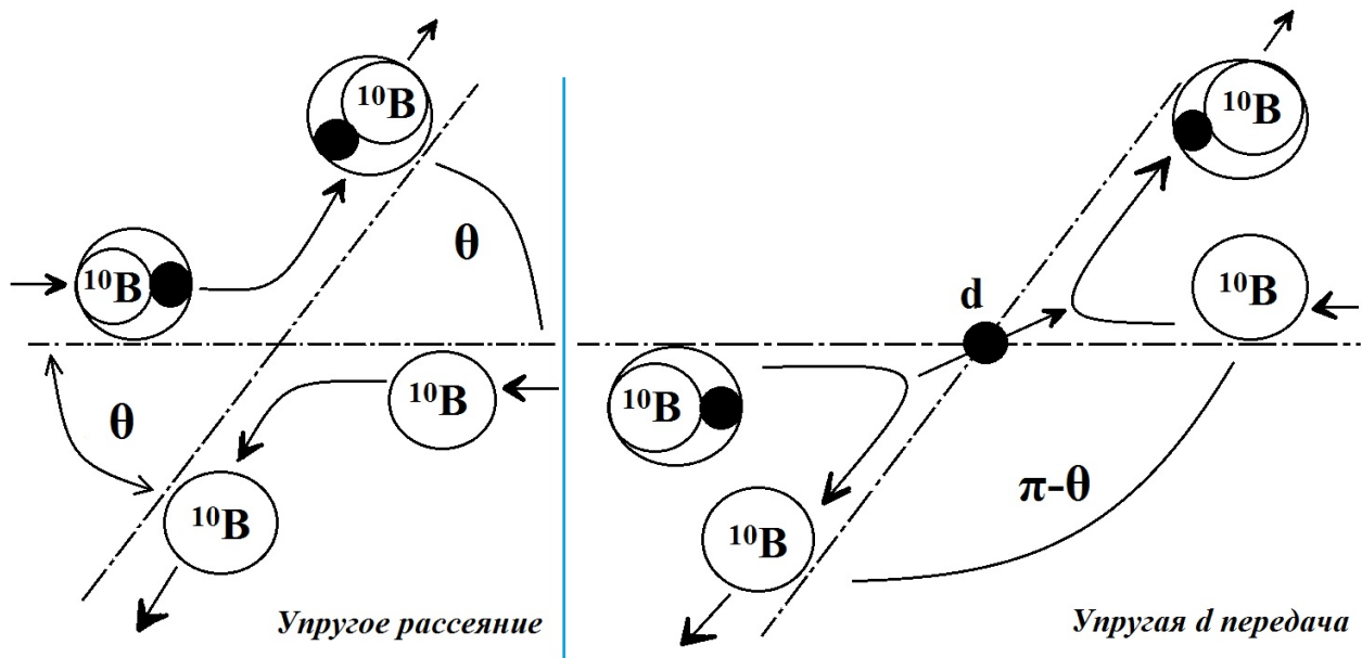
Рисунок 1 – Схематичное представление процесса упругой передачи дейтрона в реакции ^{12}\text{C} (^{10}\text{B}, ^{12}\text{C}) ^{10}\text{B}
