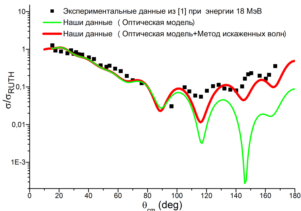
Рисунок 2 – Угловое распределение упругого рассеяния ^{10}\text{B} на ядрах ^{12}\text{C} при E_{\text{lab}}=18 МэВ [1]. Точки – эксперимент. Кривые: зеленая – расчет по оптической модели, красная – расчет с учетом обменного механизма с передачей дейтрона (FRDWBA)
